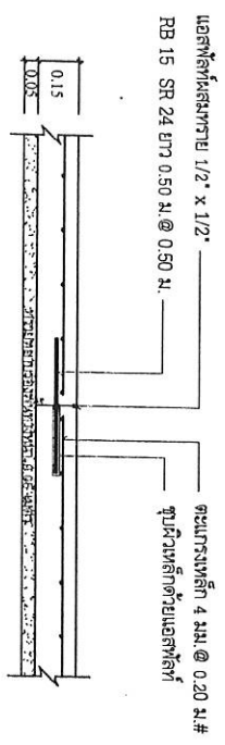
ขยาย 1 CONTRACTION JOINT ขนาดพื้นที่ 1:20
