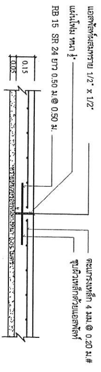
ขยาย 2 EXPANSION JOINT ขนาดพื้นที่ 1:20
